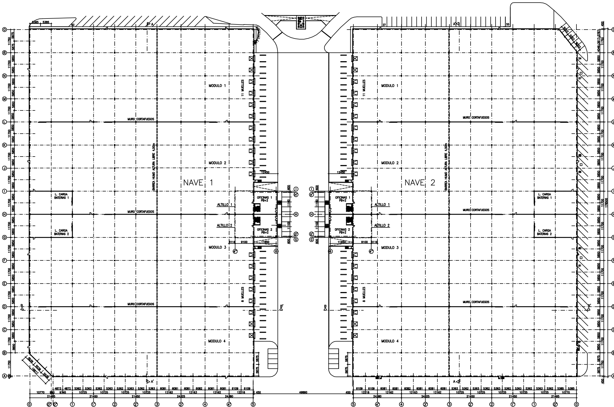
PLANTA BAJA E:1/500
