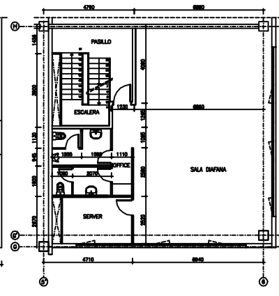
PLANTA PRIMERA E1/100 NIVEL +3850 PLANTA TIPO PARA NAVE 1
