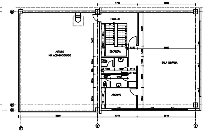
PLANTA SEGUNDA E1/100 NIVEL +7525 PLANTA TIPO PARA NAVE 1
