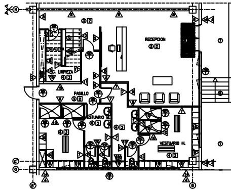
PLANTA BAJA E1/100 ACABADOS PARA NAVE 1 Y NAVE 2
