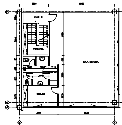
PLANTA PRIMERA E1/100 NIVEL +3850 PLANTA TIPO PARA NAVE 1
