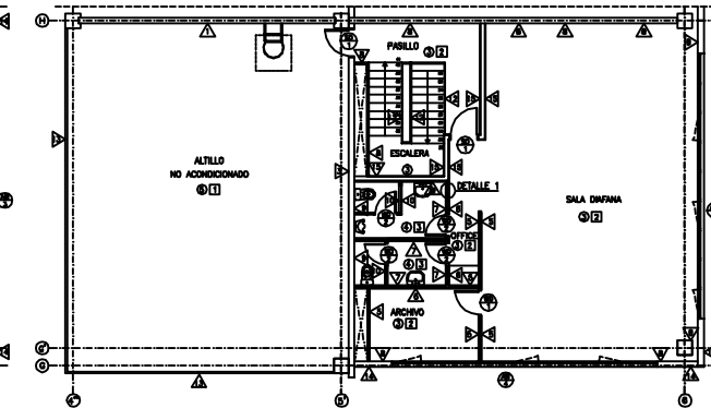
PLANTA SEGUNDA E1/100 ACABADOS PARA NAVE 1 Y NAVE 2
