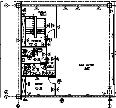
PLANTA PRIMERA E1/100 ACABADOS PARA NAVE 1 Y NAVE 2
