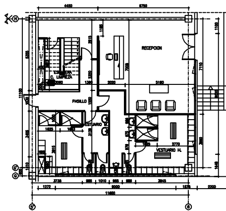
PLANTA BAJA E1/100 NIVEL ±0,00 PLANTA TIPO PARA NAVE 1 Y NAVE 2
